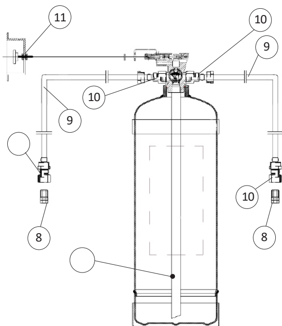
SCHEMA TIPO DI INSTALLAZIONE IMPIANTO
