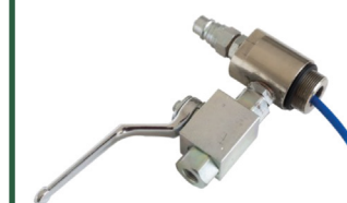
Anschlussstück für die Prüfung von tragbaren Pulver- und Schaumlöschern M30x1,5
